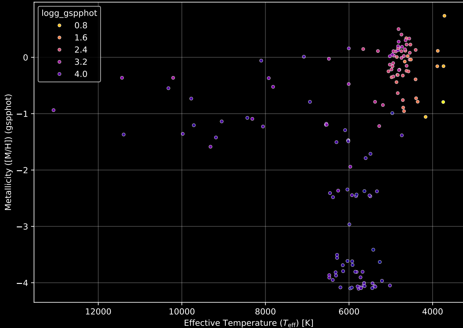
APOGEE DR17 Field: [005+05-O] Stellar Population Parameters (n= 145)
